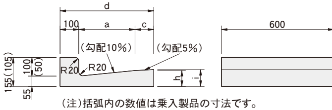
PHOTO L形側溝 1種 300
