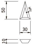
矢印詳細図(掘込式)
