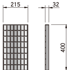
グレーチング
