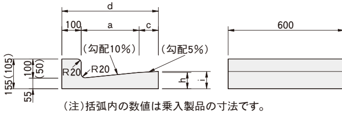
L形側溝 1種 300
