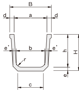
製品中央部断面図
