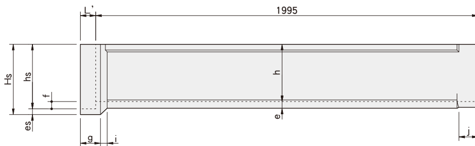
側面図
