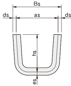
ソケット部断面図
