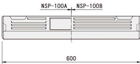
パーキングブロック NSP-100B
