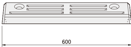
パーキングブロック ST-100
